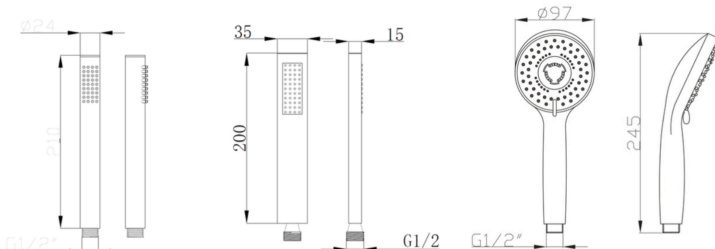
SŁUCHAWKA PRYSZNICOWA MODEL 1
