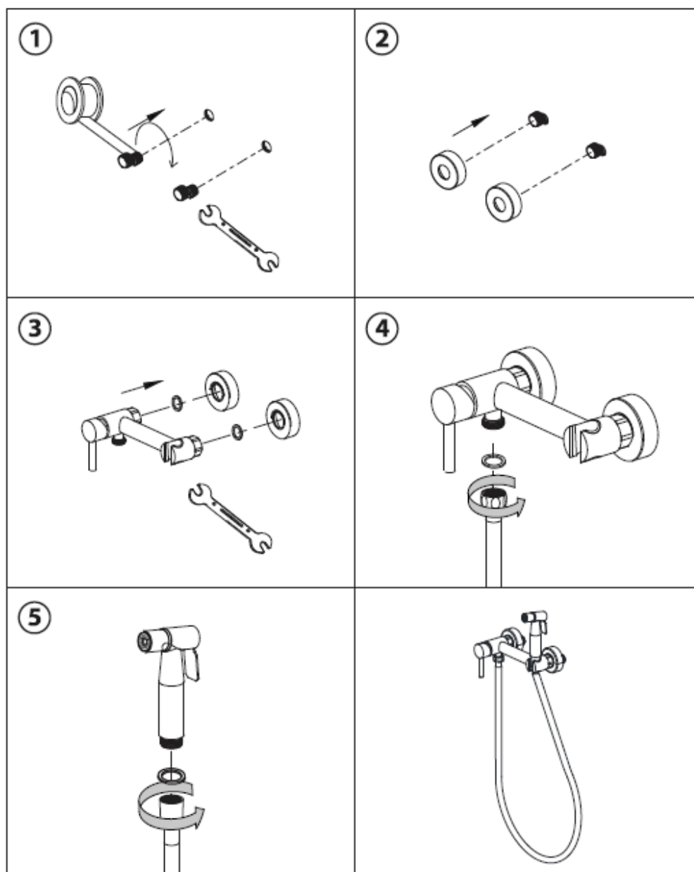
BATERIA BIDETOWA MODEL 1
