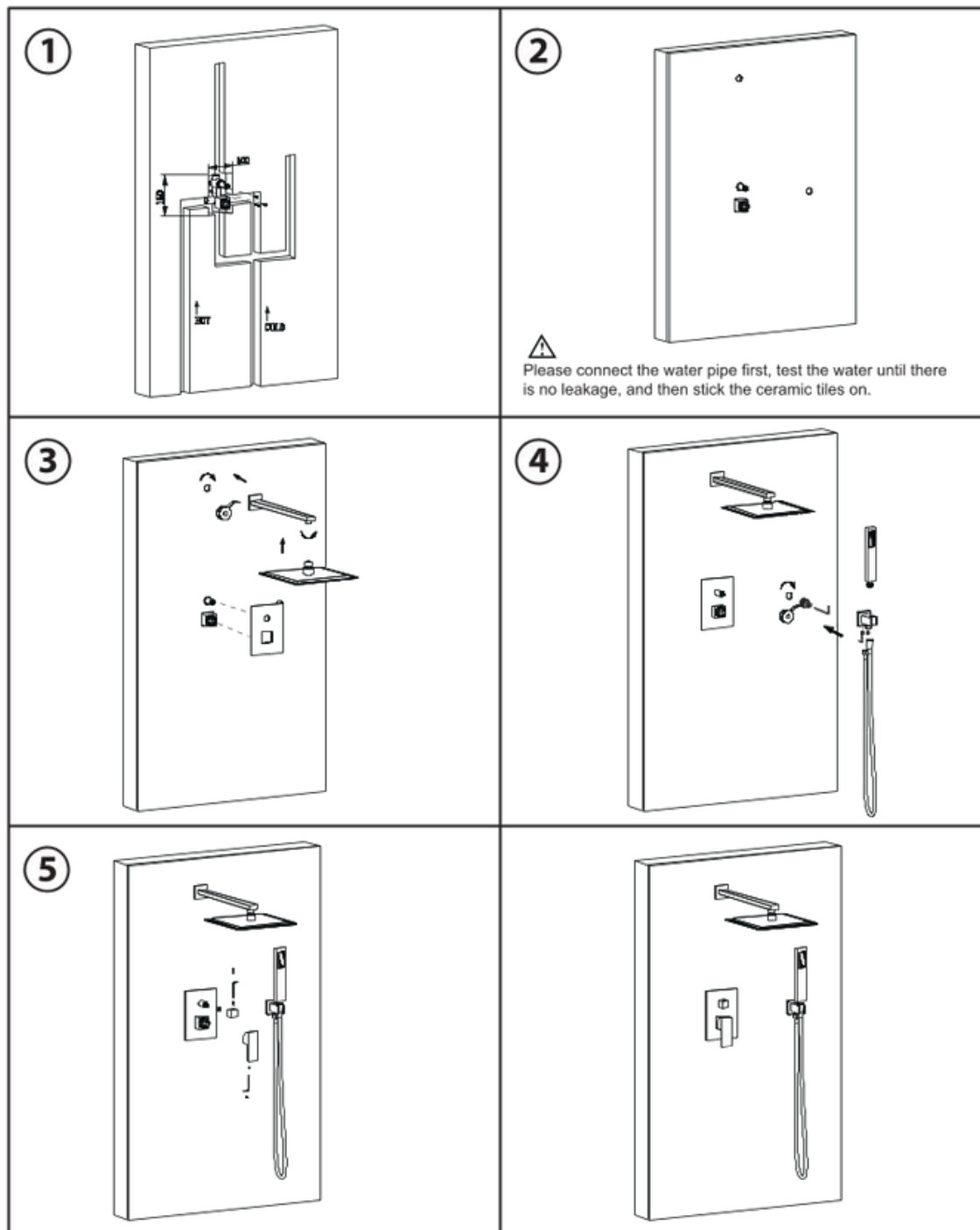
BATERIA PRYSZNICOWA MODEL 3
